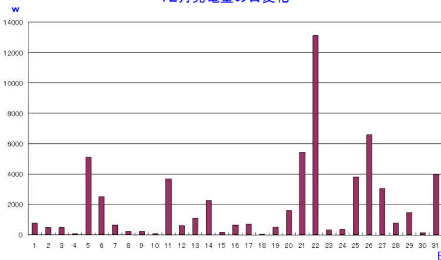
12月発電量の日変化
