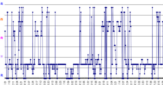
11月風向の時間変化
